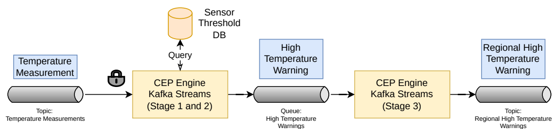
Abbildung 1: CEP Beispiel für eine Temperaturüberwachung.
